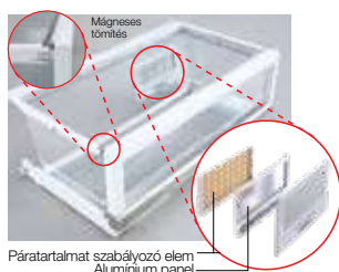
Páratartalmat szabályozó elem Alumínium panel
